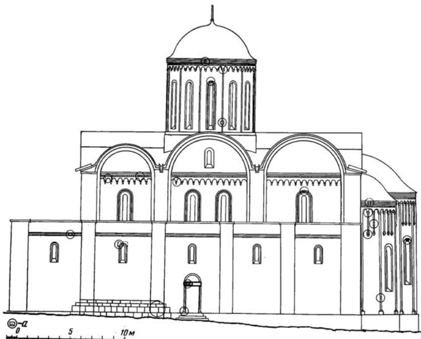
Рис. 10. Реставрація південного фасаду Успенського собору в Галичі О. Тиця: а — виявленені під час розкопок архітектурні деталі
