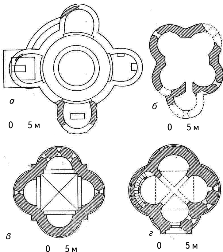
Мал. 2. План храму Святого Віта в Празькому граді (а); план церкви Святого Яна на Забродлі в Празі (б); план церкви Марії на Вавелі в Кракові (в); план церкви в Яці (г).
