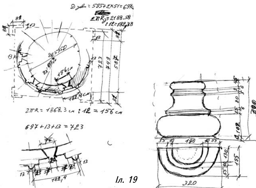
Іл. 19-23. Ескізи реконструкції церкви (за Іваном Могитичем)
